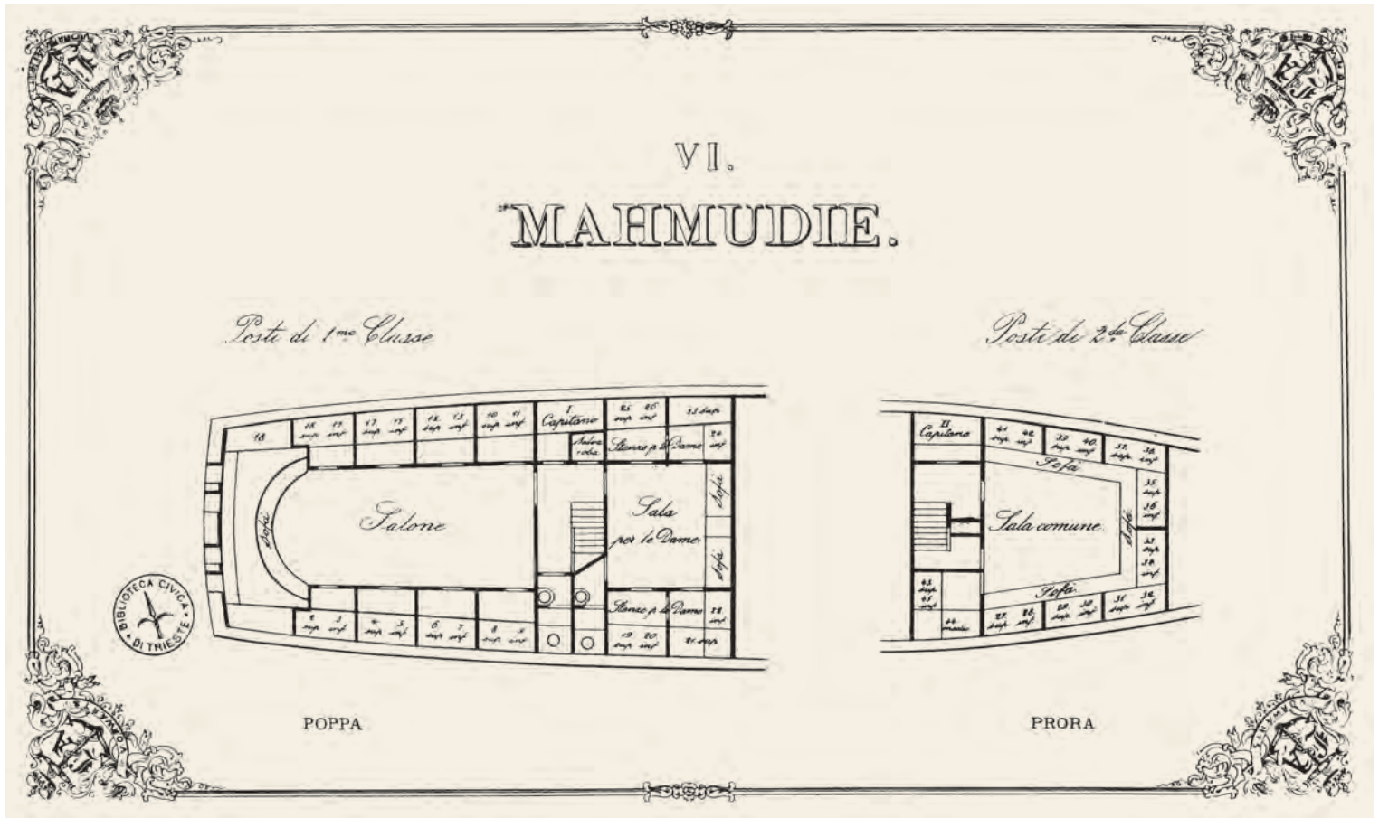
1- Lloyd'un, II. Mahmud'a ithafen Mahmudiye adı verdiği vapura ait plan (Stefani, Giuseppe, Bruno Astori, Il Lloyd Triestino: Contributo Alla Storia Italiana della Navigazione Marittima , Verona 1938, s. 114)
